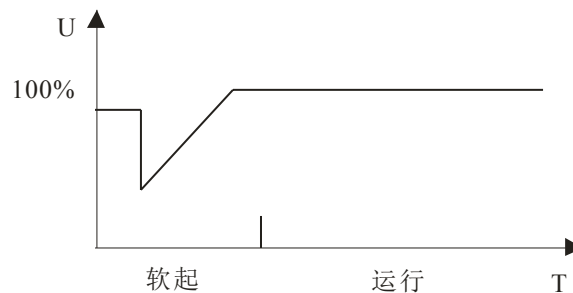
电压突跳软起动过程示意图
