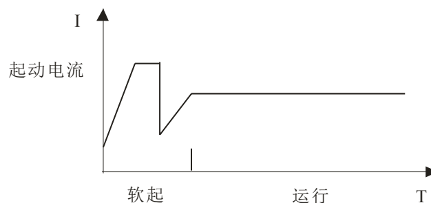
电流限流软起动过程示意图
