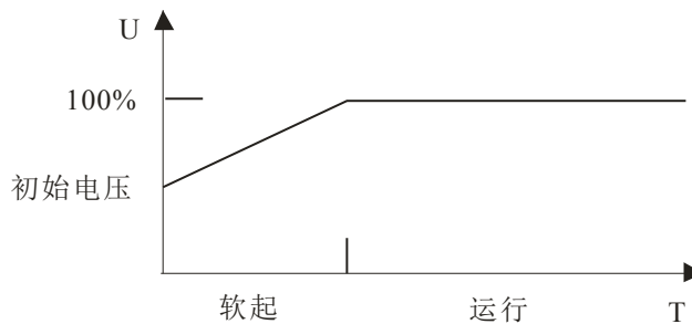
电压斜坡软起动过程示意图
